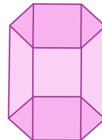
Prisme à base hexagonale
