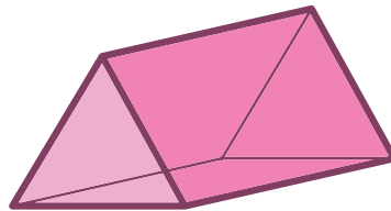
Prisme droit (prisme à base triangulaire)
