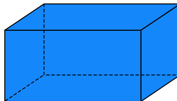
Parallélépipède (pavé droit)
