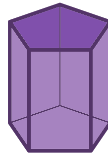
Prisme à base pentagonale
